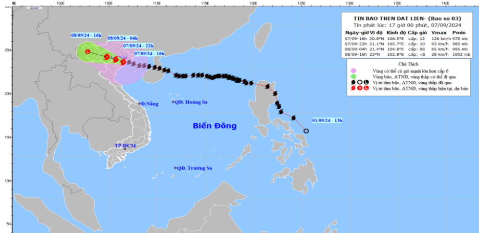
Hình 1: Bản đồ quỹ đạo và cường độ XTNĐ lúc 17h00 giờ ngày 07/09/2024
