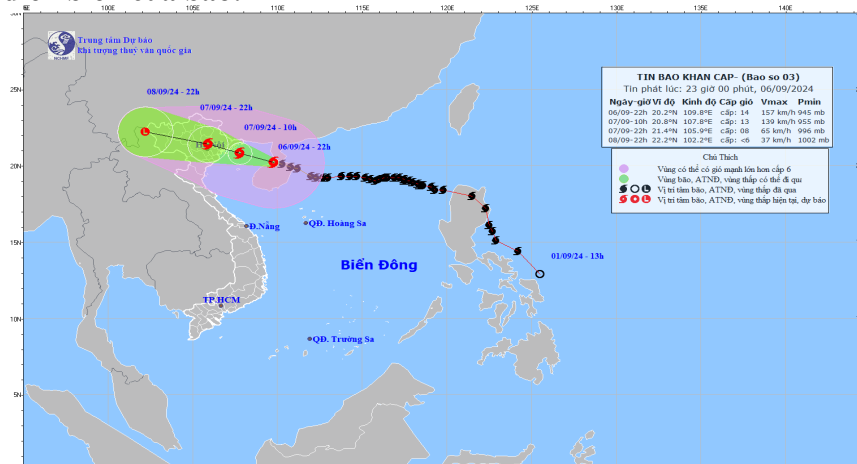
Hình 1: Bản đồ quỹ đạo và cường độ XTND lúc 23h00 giờ ngày 06/09/2024
