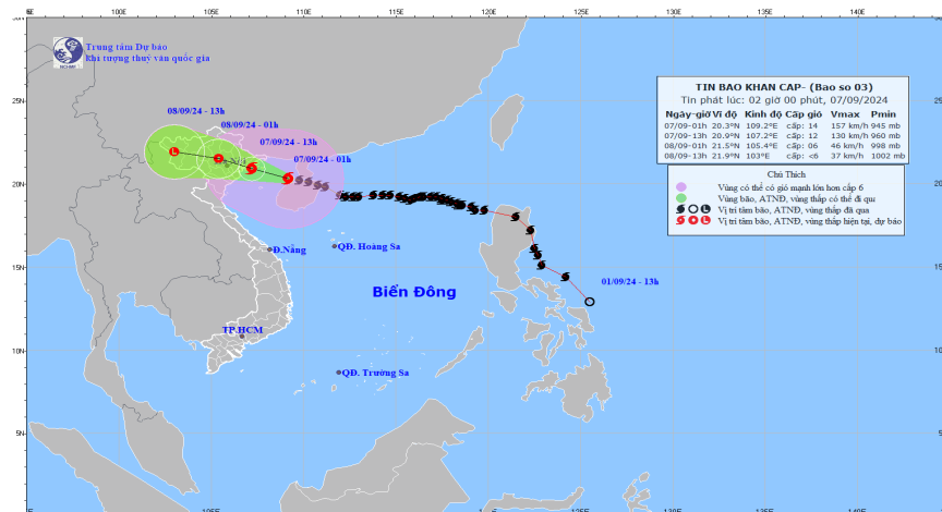
Hình 1: Bản đồ quỹ đạo và cường độ XTND lúc 02h00 giờ ngày 07/09/2024
