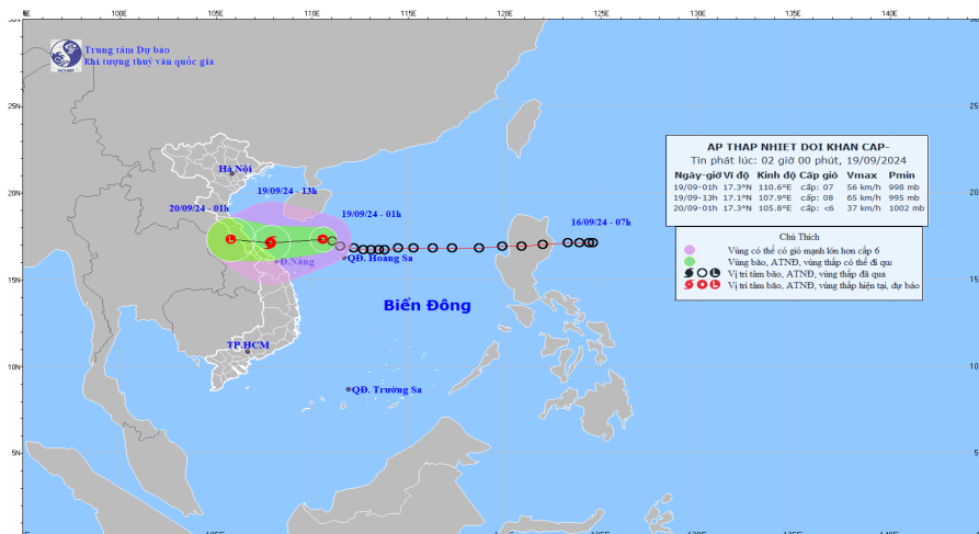
Hình 1: Bản đồ quỹ đạo và cường độ XTNĐ lúc 02h00 giờ ngày 18/09/2024
